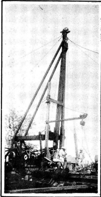
Equipo perforando en Motembo.
