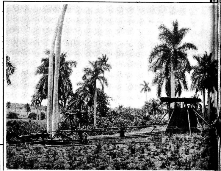
Pozo numero 4, de Bacuranao, perforado en 1917. Actualmente está dando petróleo.
